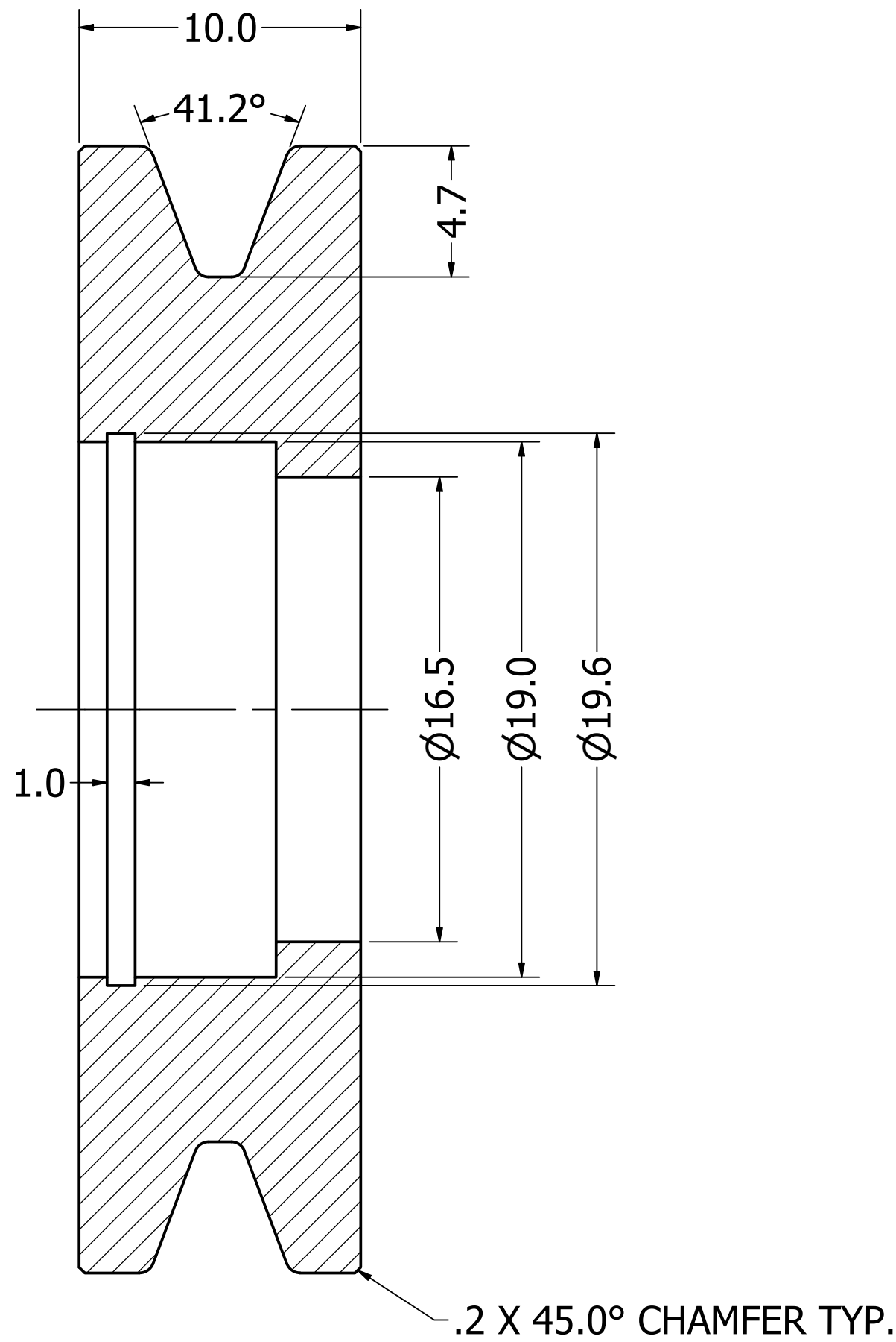
SECTION A-A SCALE 5 : 1
